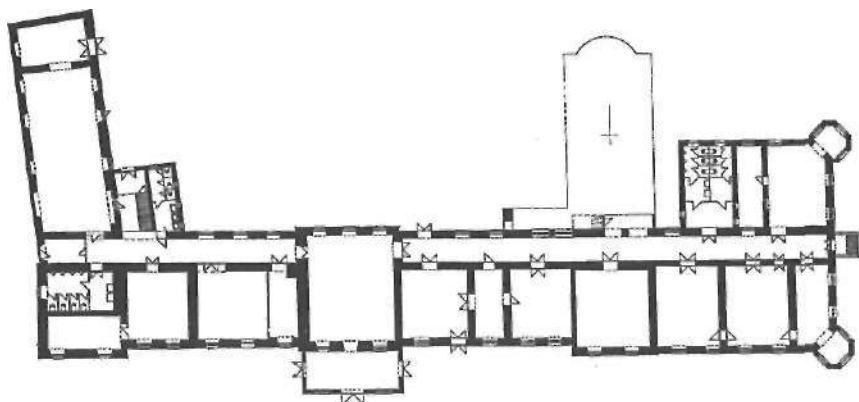
Barokový kaštieľ Ladce - pôdorys prízemí
