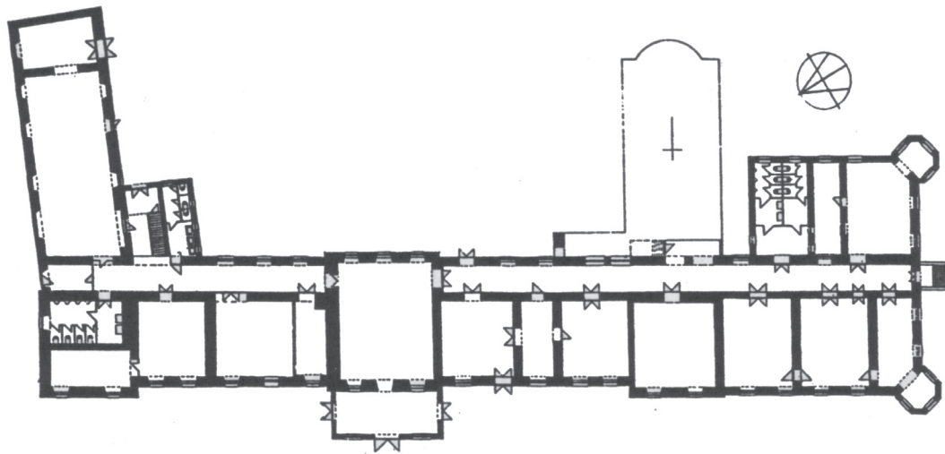
Kaštieľ - pôdorys prízemia
